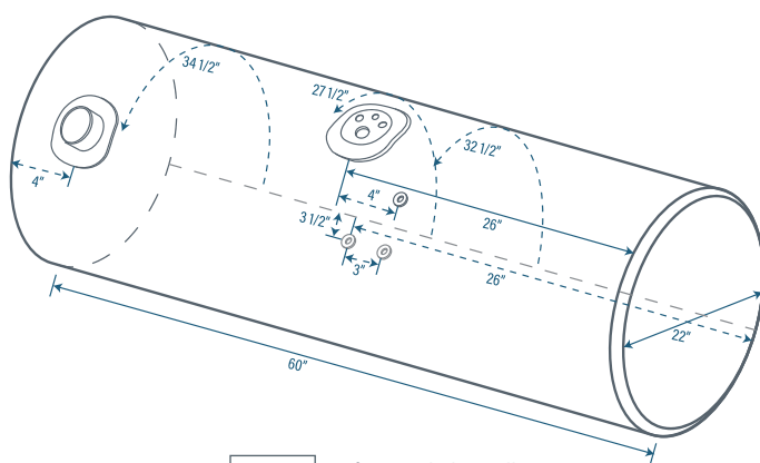
TAT3GAT Tapón atrás lado copiloto 378.5 Litros / 100 Galones Aluminio liso calibre 14 Aleación: 5052 H32
