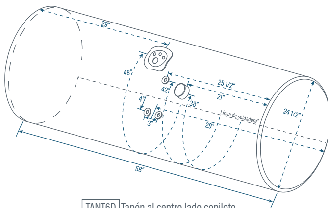
TANT6D Tapón al centro lado copiloto
