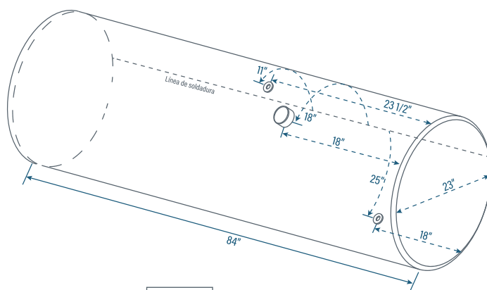
TANFL58D Sin flotador
