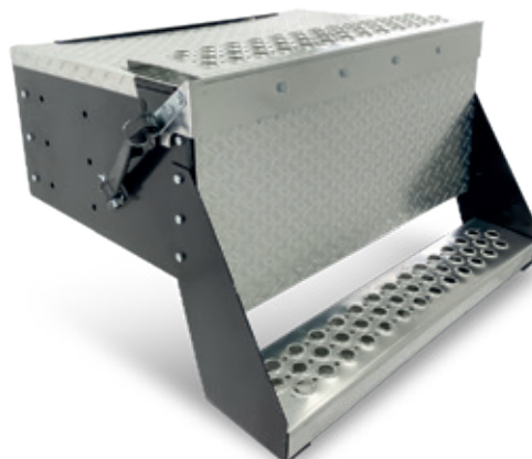
ALUE2 Caja de batería/estribo T-370 modelo nuevo (2003 o posteriores)
