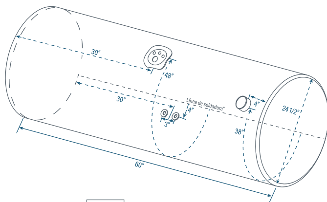
TANK45D Tapón adelante lado copiloto
