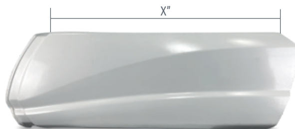
LH X FAL064L Cubretanque central s/ext fibra de vidrio 55" FAL066L Cubretanque central s/ext fibra de vidrio 62.5" FAL068L Cubretanque central s/ext fibra de vidrio 67.5"
