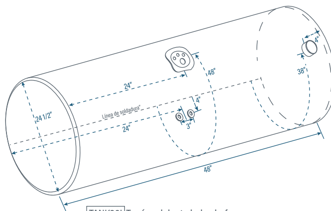
TANK36I Tapón adelante lado chofer
