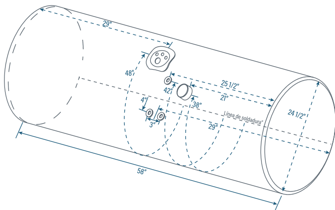
TANT6D Tapón al centro lado copiloto
