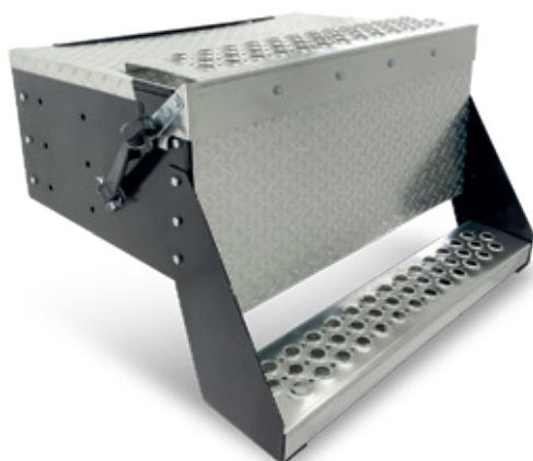
ALUE2 Caja de batería/estribo T-300 modelo nuevo (2003 o posteriores)
