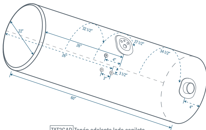
TAT3GAD Tapón adelante lado copiloto 378.5 Litros / 100 Galones Aluminio liso calibre 14 Aleación: 5052 H32
