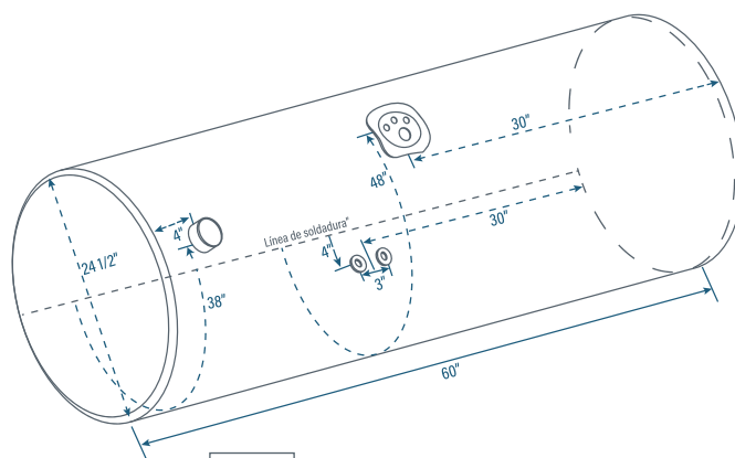
TANK45I Tapón adelante lado chofer
