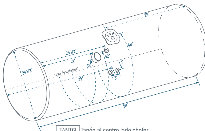
TANT6I Tapón al centro lado chofer
