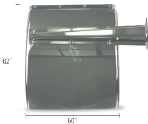
CZL0501 Zoquetera torton, cromo sujeción placa
