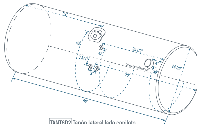
TANT6D2 Tapón lateral lado copiloto
