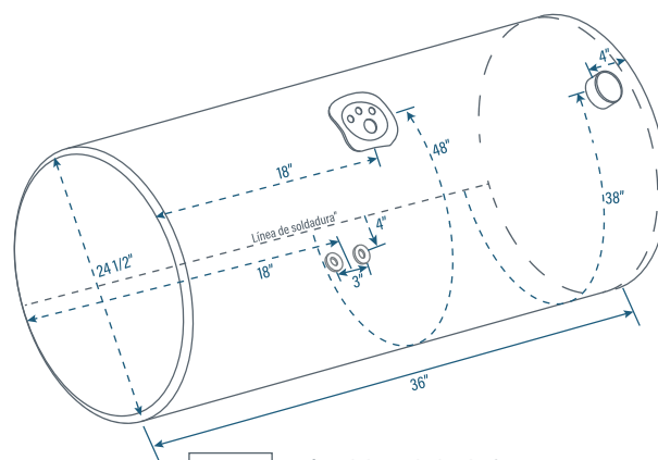
TANK28I Tapón adelante lado chofer
