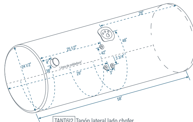
TANT6I2 Tapón lateral lado chofer
