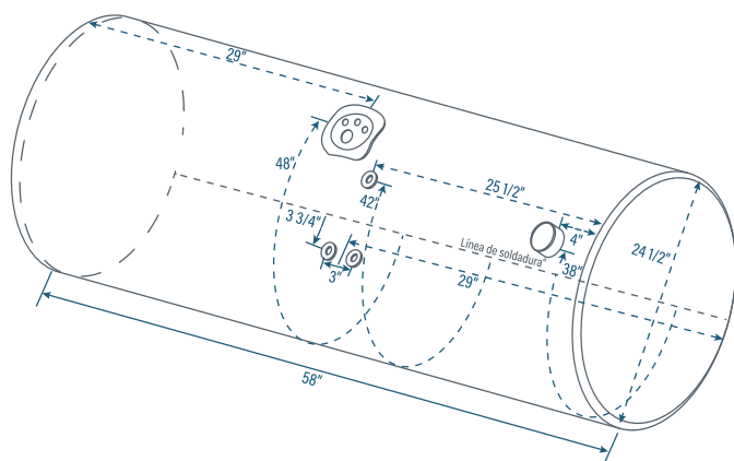
TANT6D2 Tapón lateral lado copiloto
