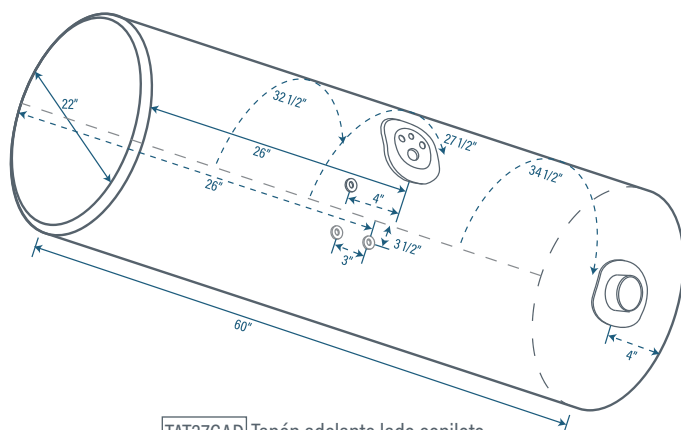
TAT37GAD Tapón adelante lado copiloto 378.5 Litros / 100 Galones Aluminio liso calibre 14 Aleación: 5052 H32
