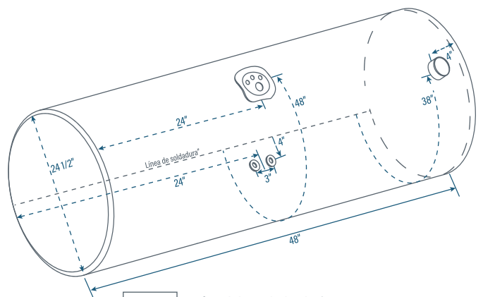
TANK36L Tapón adelante lado chofer
