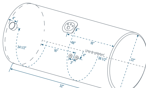
TAT3CAT Tapón atrás lado copiloto 208 Litros / 55 Galones Aluminio liso calibre 14 Aleación: 5052 H32
