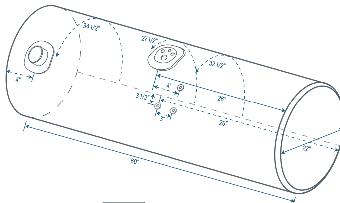
TAT37GAT Tapón atras lado copiloto 378.5 Litros / 100 Galones Aluminio liso calibre 14 Aleación: 5052 H32
