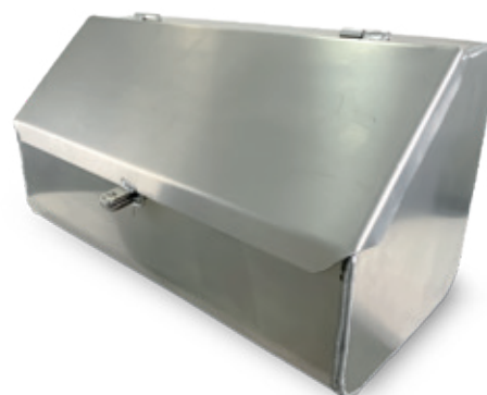
CCH00311 Caja herramienta Aluminio Liso 22" X 12" X 12"
