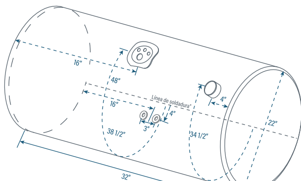
TAT3CAD Tapón adelante lado copiloto 208 Litros / 55 Galones Aluminio liso calibre 14 Aleación: 5052 H32
