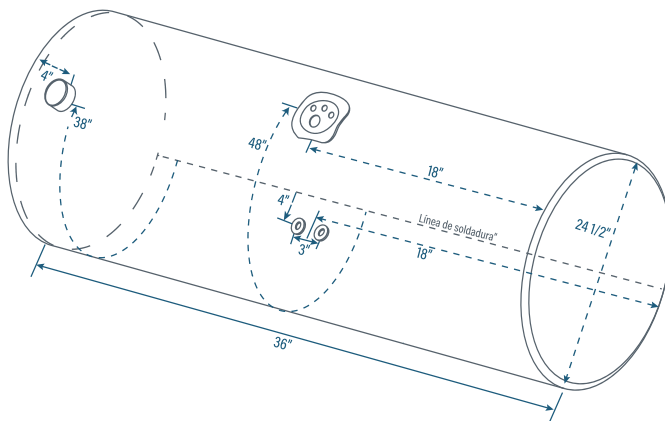
TANK28D Tapón adelante lado copiloto
