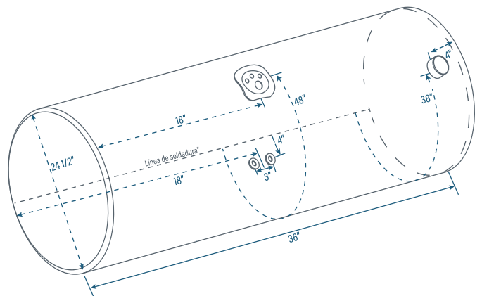
TANK28L Tapón adelante lado chofer
