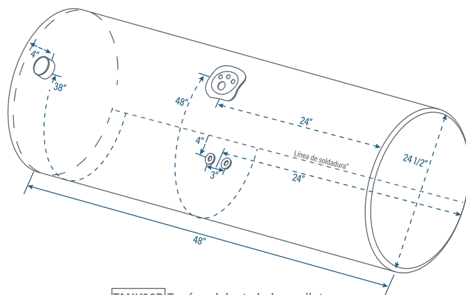
TANK36D Tapón adelante lado copiloto
