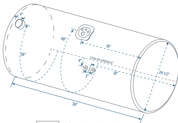
TANK36D Tapón adelante lado copiloto
