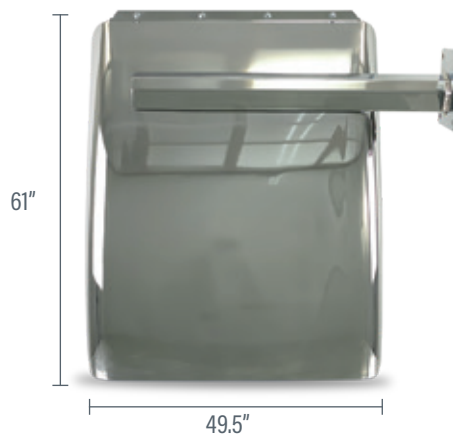
CZL0453 Camión 3 toneladas cromo sujeción placa
