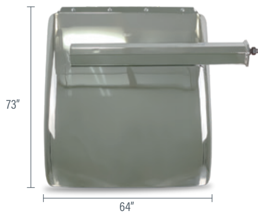
CZL0806 Tipo americano cromo sujeción placa
